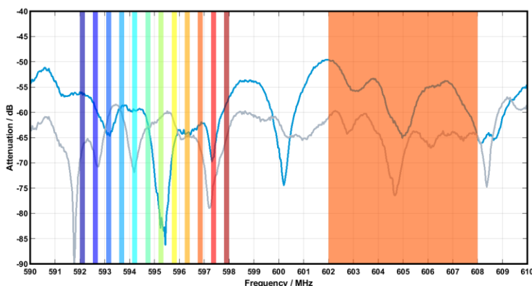
TV-Kanalnutzung (6 MHz) mehrerer Schmalbandsysteme (links) und eines WMAS (rechts), das Zeitslots anstelle von festen Frequenzen zuweist. Die blauen und grauen Linien sind die Dämpfung (in dB) des gemessenen Empfangssignals an den Beispielantennen 1 und 2
